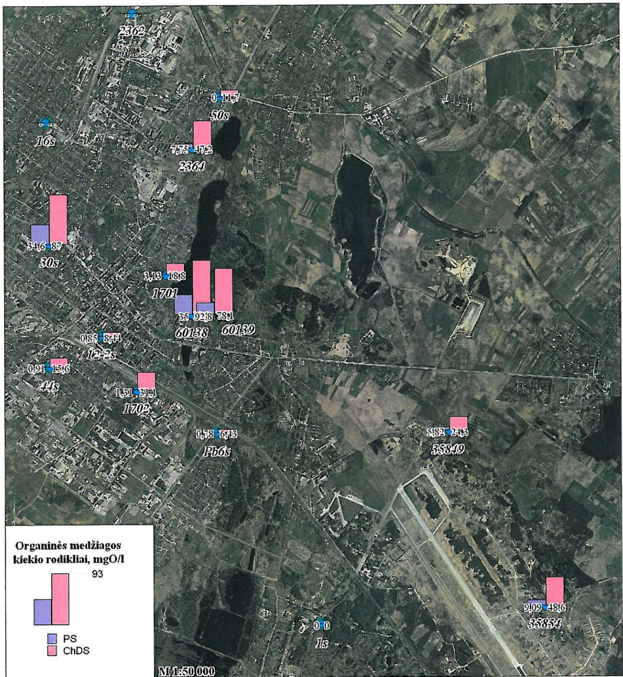
7 pav. Permanganato indekso ir ChDS vertės gruntiniame vandenyje (2017 m. ruduo)
