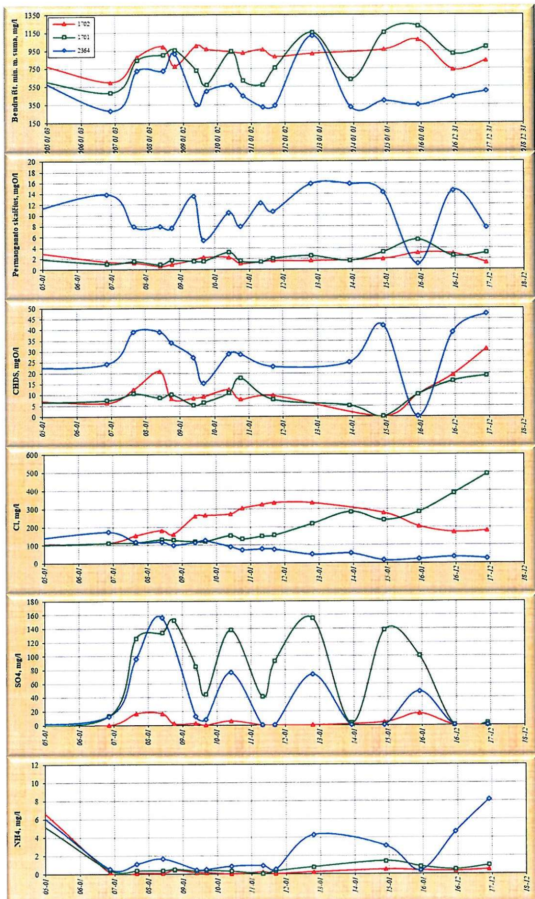
9 pav. Gręžinių gruntinio vandens cheminės sudėties rodiklių kaita (2005–2017 m.)
