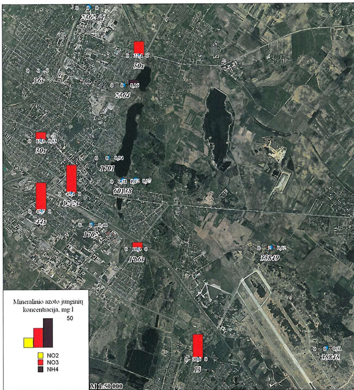
8 pav. Mineralinio azoto koncentracija gruntiniame vandenyje (2017 m. ruduo)
